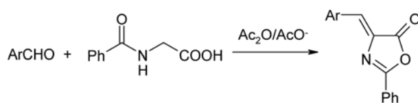
Fig. 7: Erlenmeyer–Plöchl synthesis.
